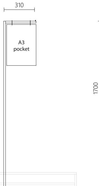
L stand POS 1x A3
