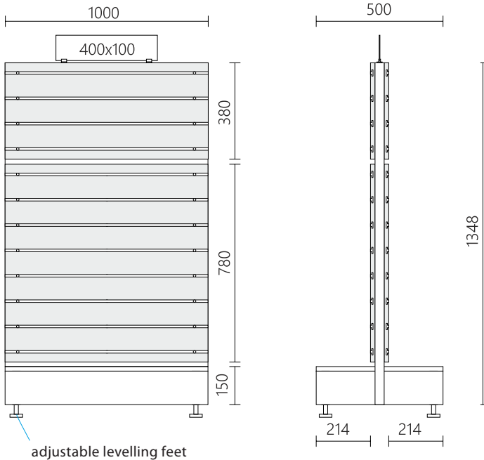
Impulse gondola module
