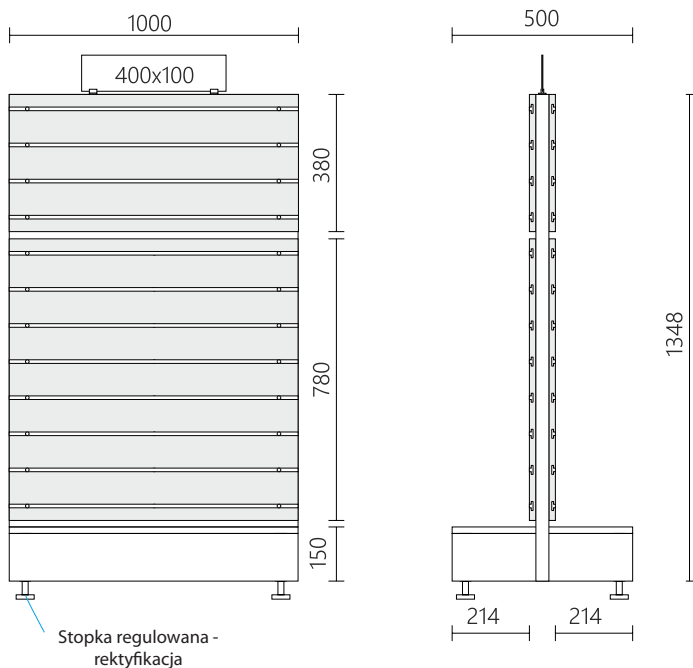
Moduł gondoli zakupów impulsowych
