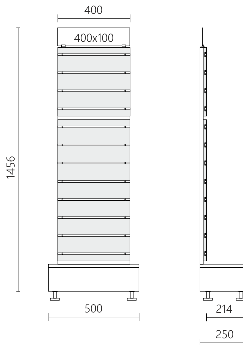
Płyta gondoli zakupów impulsowych
